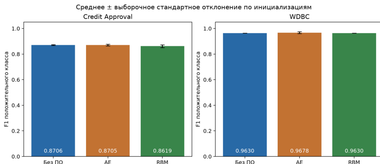
Рисунок 6 — Средний F1 и его разброс по трём инициализациям
