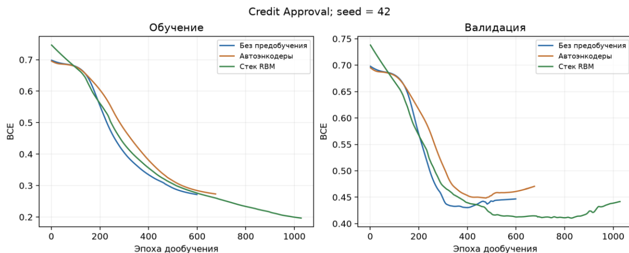
Рисунок 2 — Обучение и валидация Credit Approval при seed 42
