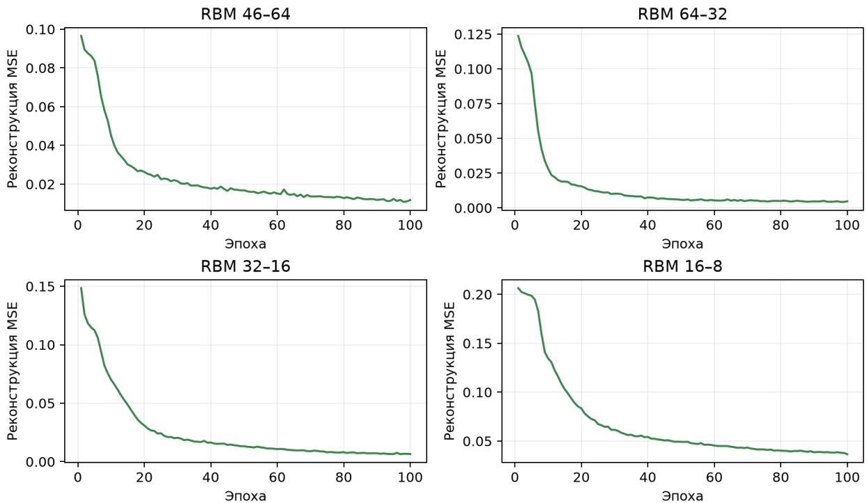
Рисунок 1 — Диагностическая реконструкция четырёх RBM Credit Approval
