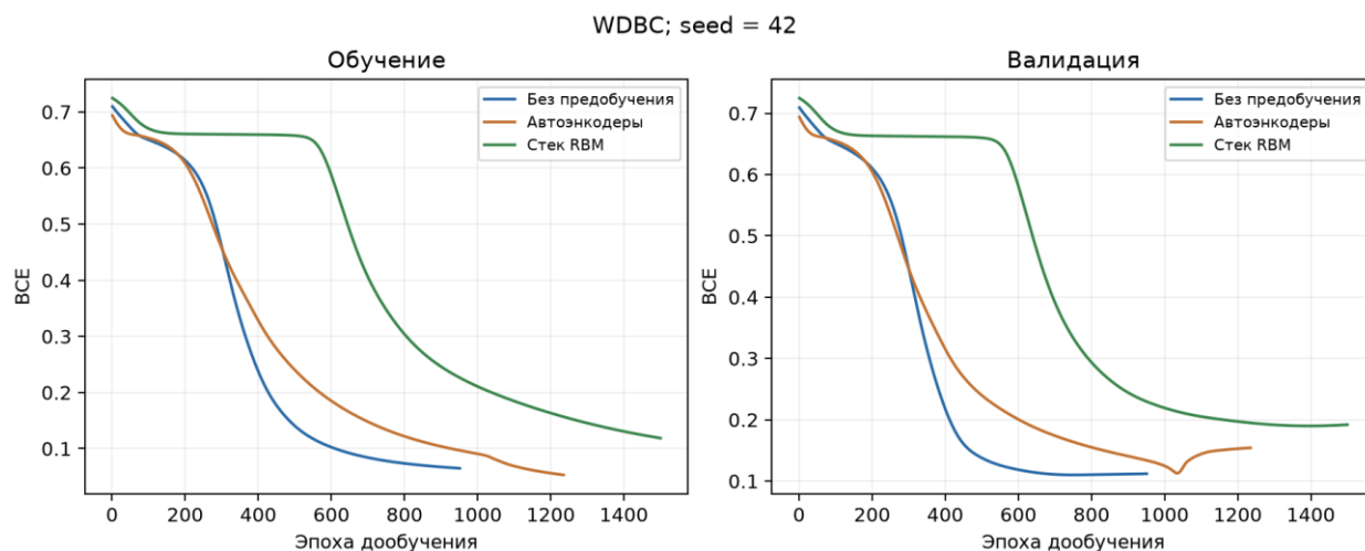
Рисунок 4 — Обучение и валидация WDBC при seed 42
