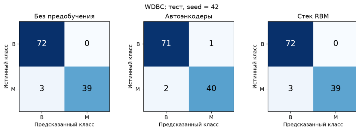
Рисунок 5 — Матрицы ошибок WDBC на тесте при seed 42
